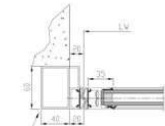
Mindest-Auflage auf Seitenwand = 35mm dokalA Anfahr60_20s
