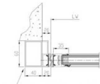
Mindest-Auflage auf Seitenwand = 35mm dokalA Anfahr60_20s
