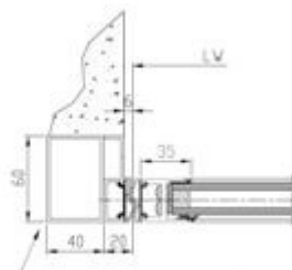
Mindest-Auflage auf Seitenwand = 35mm dokalA Anfahr60_6s
