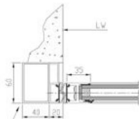
Mindest-Auflage auf Seitenwand = 35mm dokalA Anfahr60_0s
